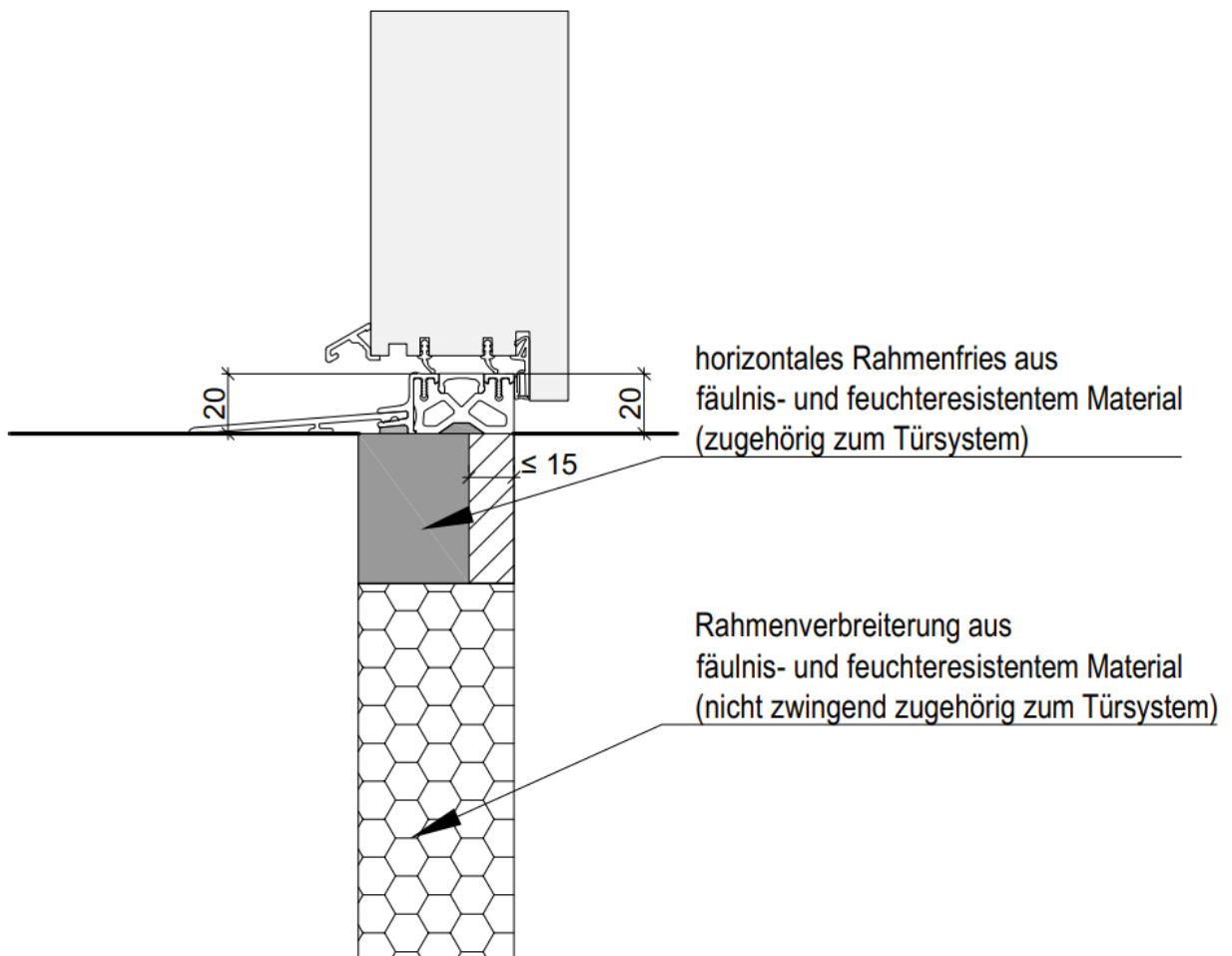
Abbildung nur schematisch, ohne Abdichtungsanschlüsse dargestellt
